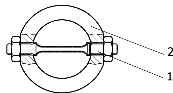
1 - образец; 2- приспособление
