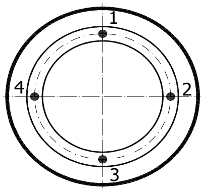
Рисунок Г.3 - Схема расположений точек, в которых должны производиться измерения толщины образца
